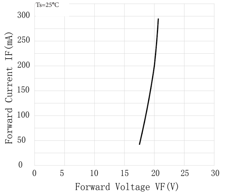
V_f ----- I_f
